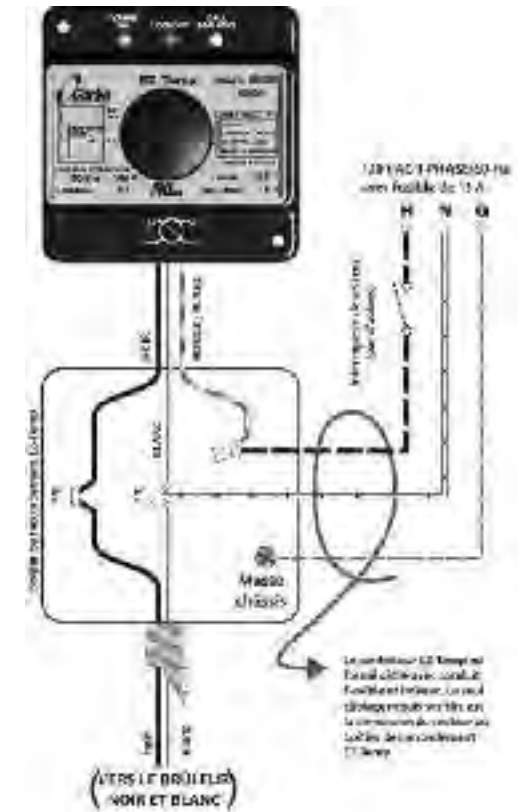
FIGURE 5 : Brûleur Beckett ou Wayne avec Carlin EZ-Temp Pour les modèles : 32, 33, 50, 51, 120
